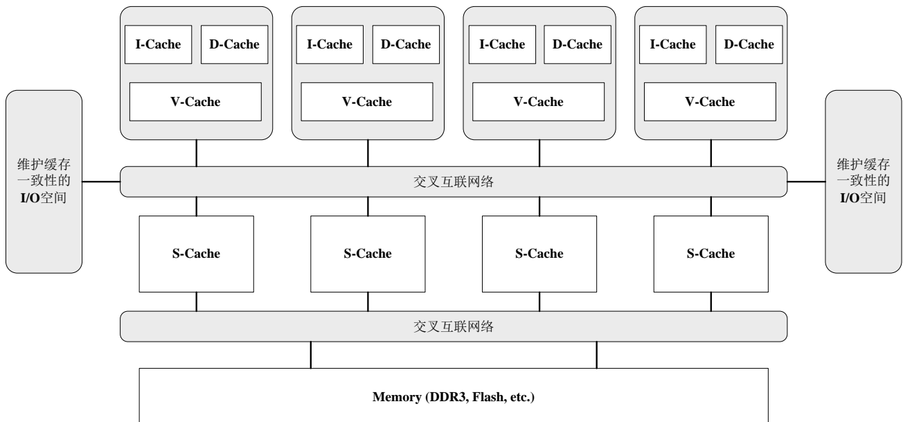
图 5-1 龙芯 3A3000 芯片处理器存储层次
