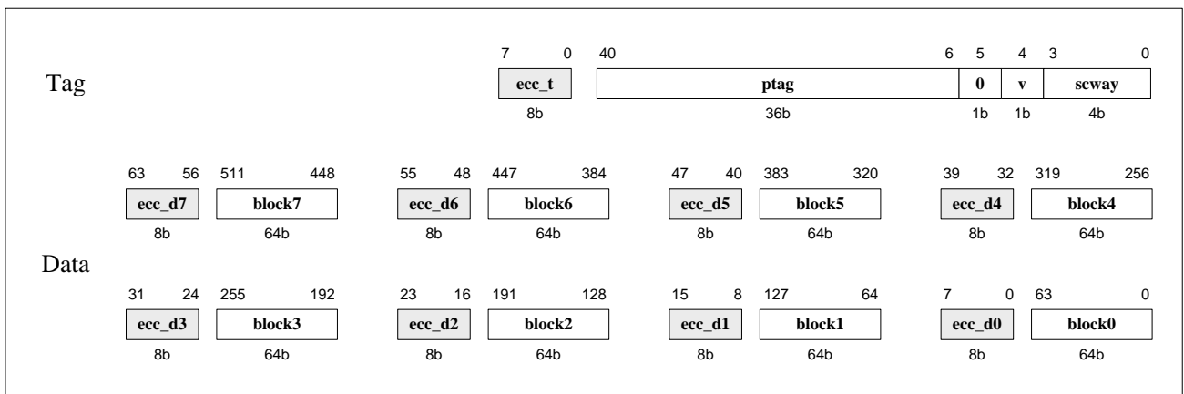
图 5-2 一级指令缓存行结构示意图
