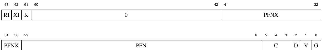
图 7-3 EntryLo0 和 EntryLo1 在 DMFC0/DMTC0 指令访问时的寄存器格式
