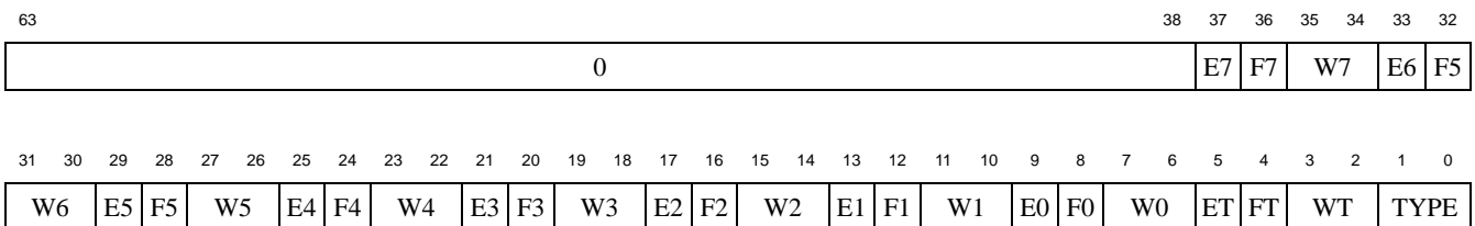
图 7-47 CacheErr 寄存器用于 D-Cache 校验错信息时的格式
