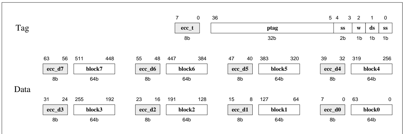
图 5-5 三级共享缓存行结构示意
