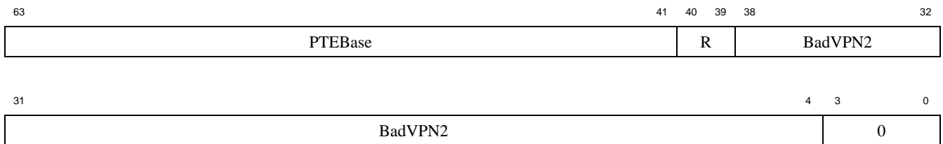
图 7-38 XContext 寄存器格式
